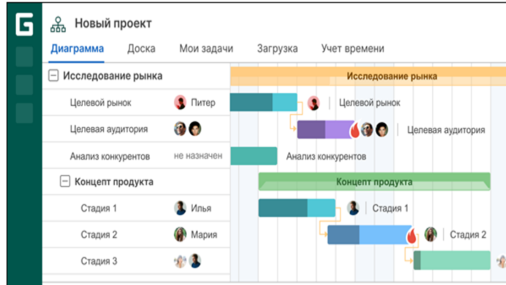
GanttPRO
