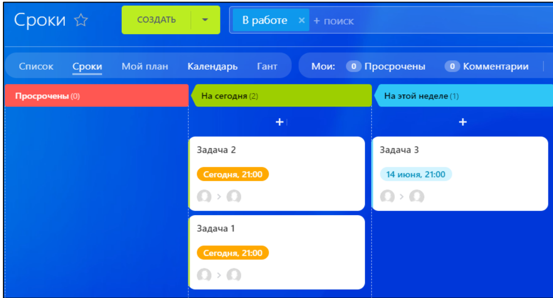
Bitrix24
