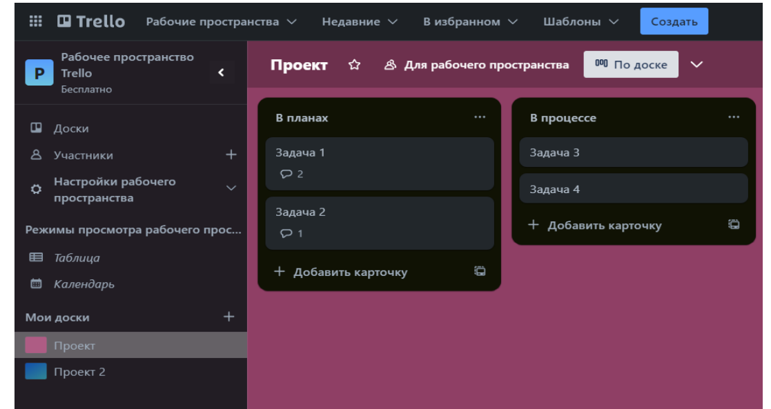
Trello
